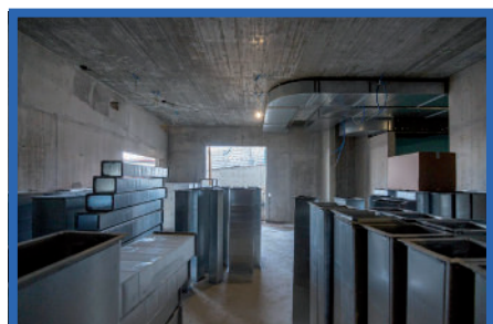
POSE DE LA VENTILATION
