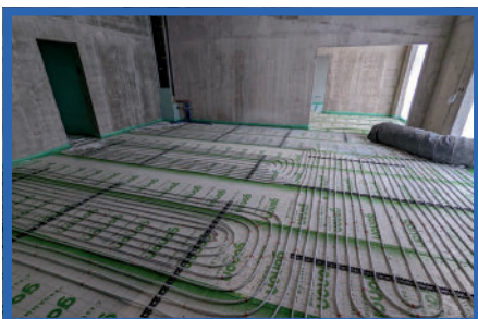
BOUCLES DE CHAUFFAGE AU REZ INFÉRIEUR
