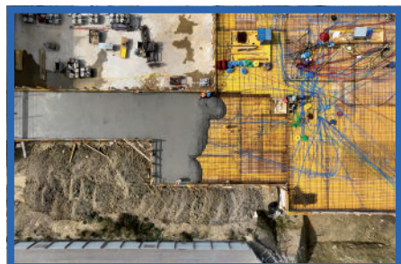
COULAGE DU REZ SUPÉRIEUR
